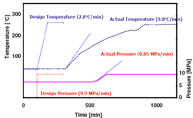
(b) Actual Transient
